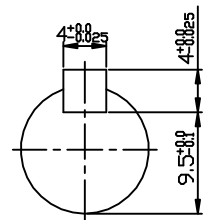
INPUT SHAFT
