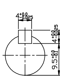
INPUT SHAFT
