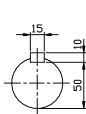
INPUT SHAFT
