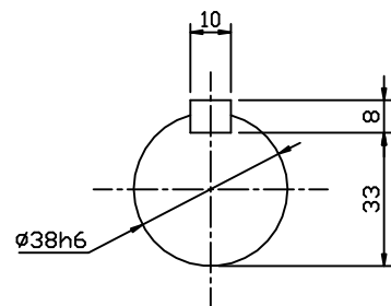
INPUT SHAFT
