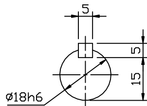
INPUT SHAFT
